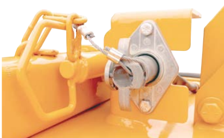
Accès au disque rapide et sans outil, avec 2 sécurités : une électrique et l'autre mécanique.
